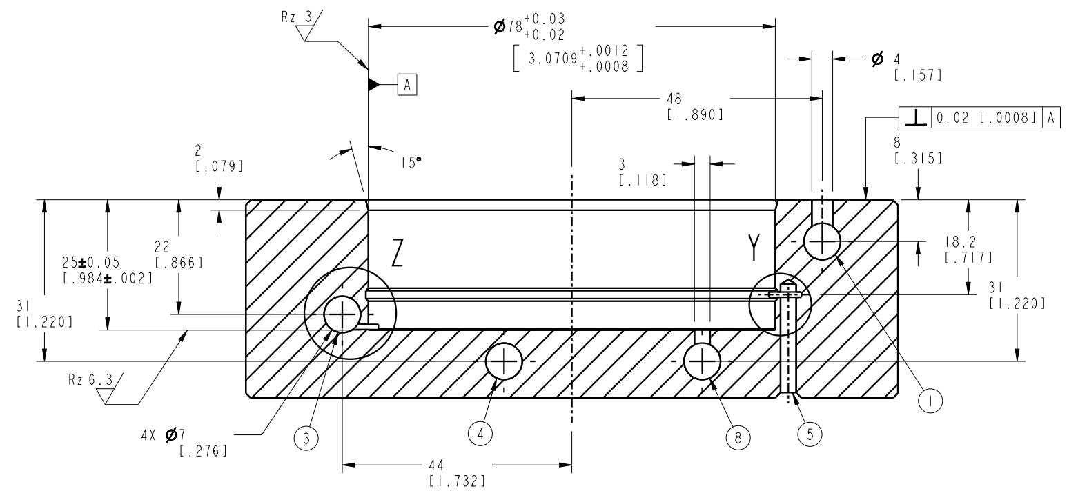
SECTION A-A
