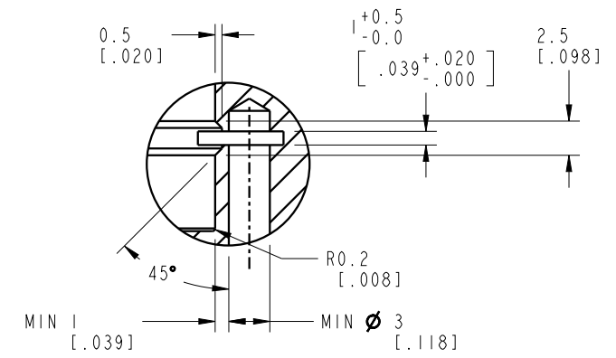
DETAIL Y
