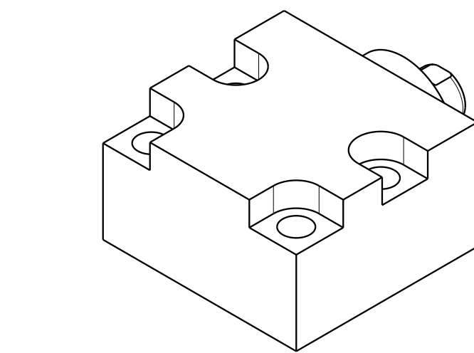
ILC25120820 REV A ECN 5974 SCALE 1.000
