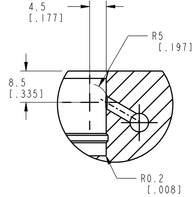
DETAIL Y
