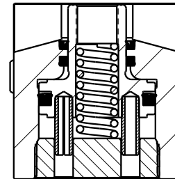
SECTION A-A SCALE 0.500
